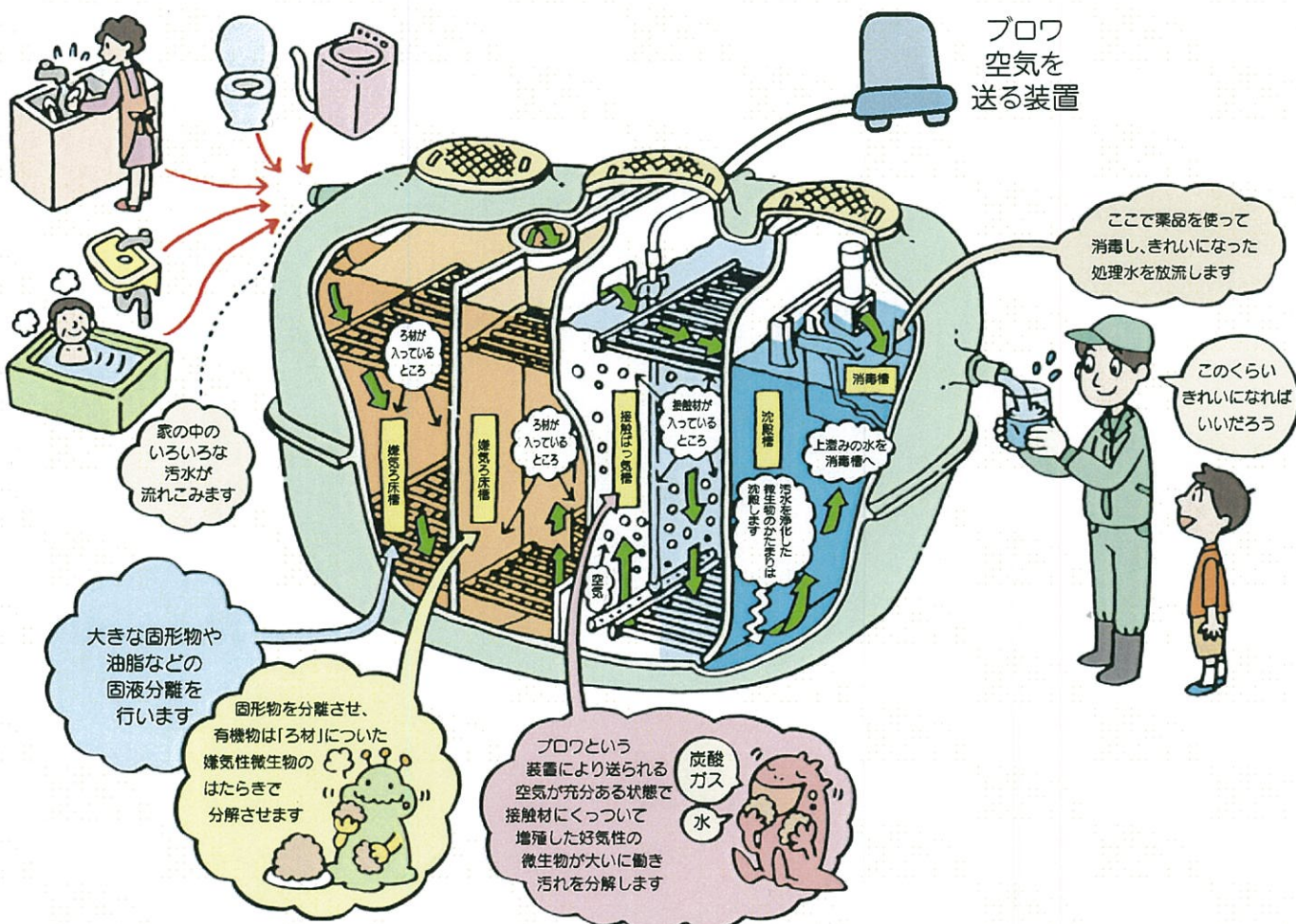
嫌気ろ床接触ばっ気方式の場合
